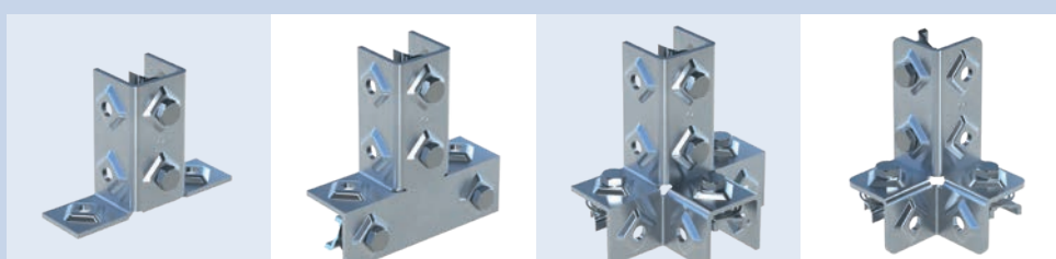
Kutna spojnica EV CC 41-2 W
